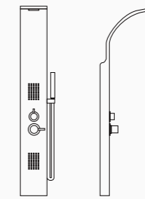
RL-P217W 1455*200*70mm Top Part 450mm
